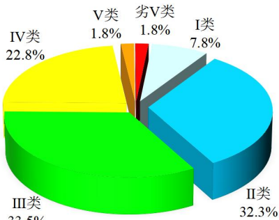
图1 2025年6月全省地表水水质类别比例图
