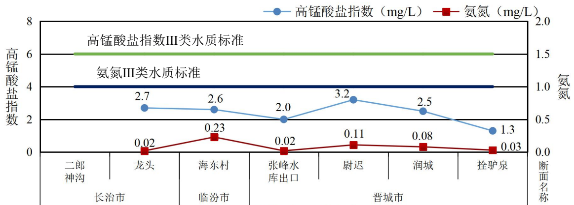
图4 沁河高锰酸盐指数、氨氮浓度沿程变化
