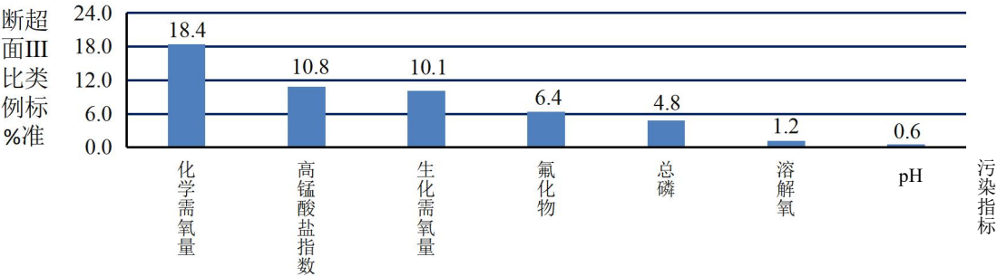
图2 2025年6月全省地表水污染指标统计
