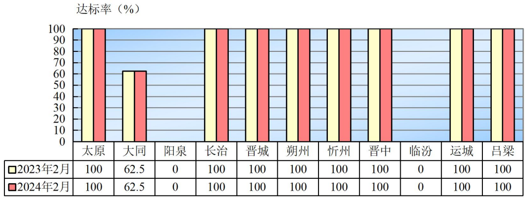
图1 山西省地级市饮用水源地水质达标率情况
